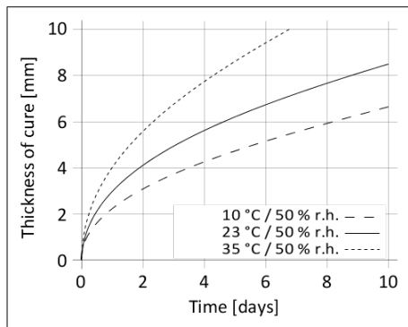
グラフ 1: Sikaflex®-554 の硬化速度
