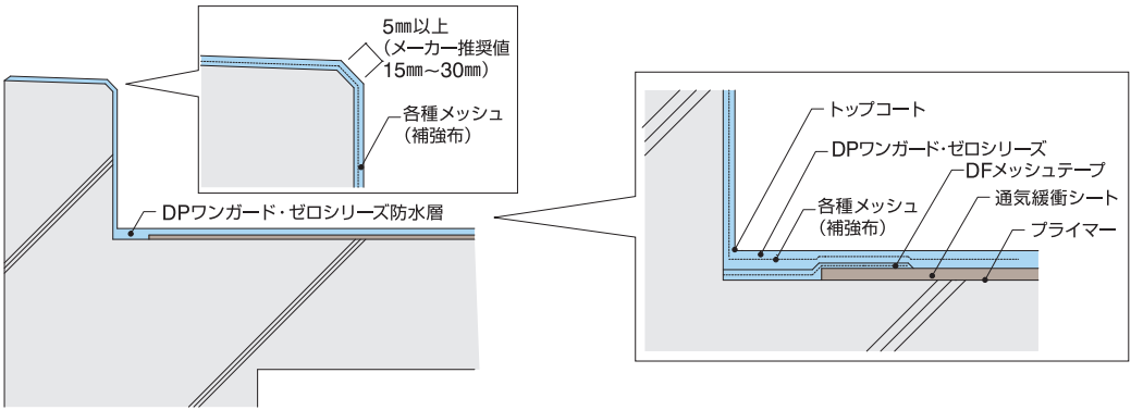
パラペット タイル取り合い
