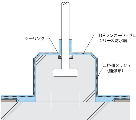
フェンス基礎
