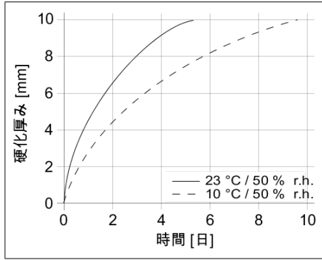
グラフ 1: Sikaflex®-298の硬化速度
