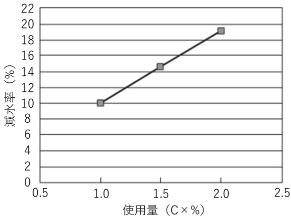
使用量と減水率の関係
