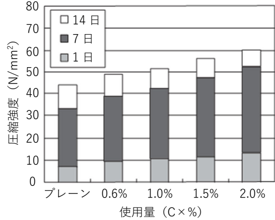
使用量と圧縮強度
