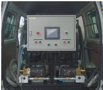
圧送機本体
