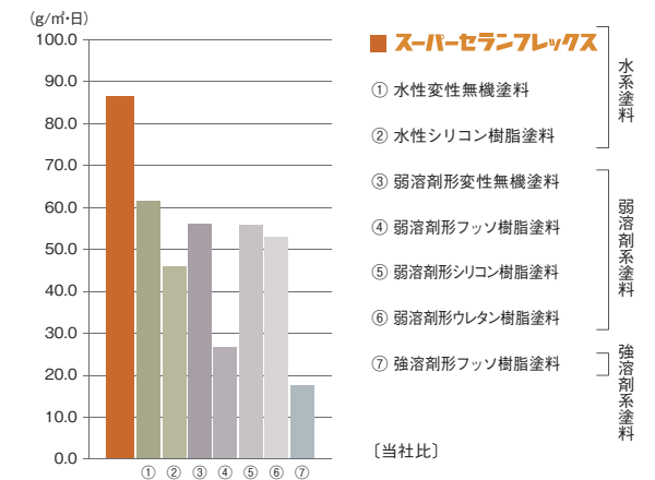
JIS Z 0208 透湿度試験結果 (A法: 25°C90%による)
