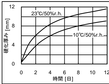
グラフ 1: Sikaflex®-251 の硬化速度
