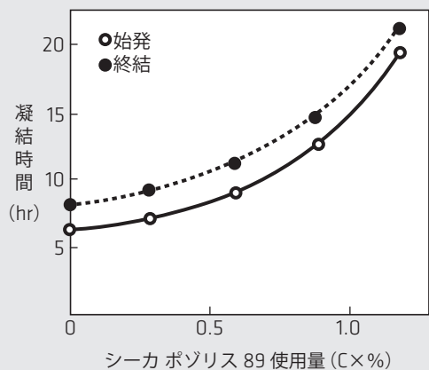
使用量と凝結時間の関係
