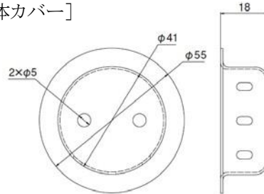
[本体カバー]
