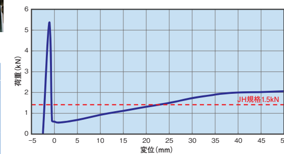
押抜き試験 (変位荷重曲線イメージ)
