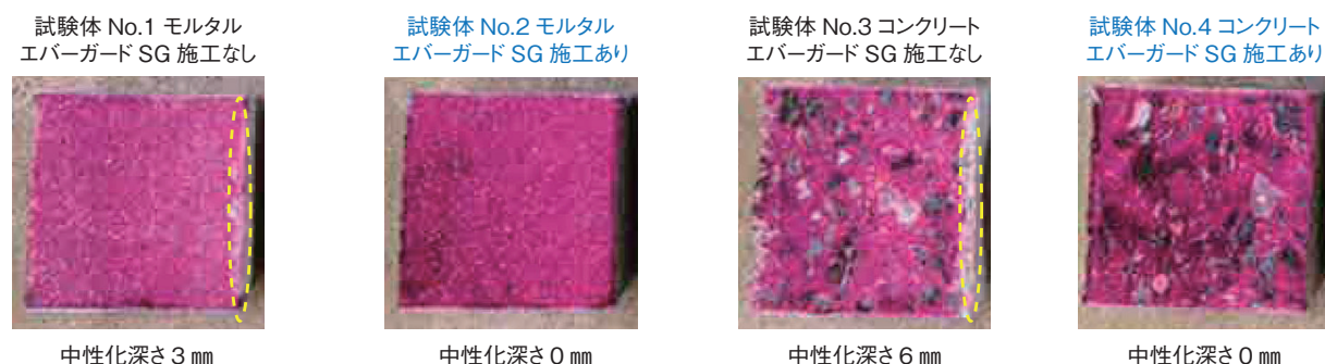
試験体 No.1 モルタル エバーガード SG 施工なし 中性化深さ 3 mm 試験体 No.2 モルタル エバーガード SG 施工あり 中性化深さ 0 mm 試験体 No.3 コンクリート エバーガード SG 施工なし 中性化深さ 6 mm 試験体 No.4 コンクリート エバーガード SG 施工あり 中性化深さ 0 mm
